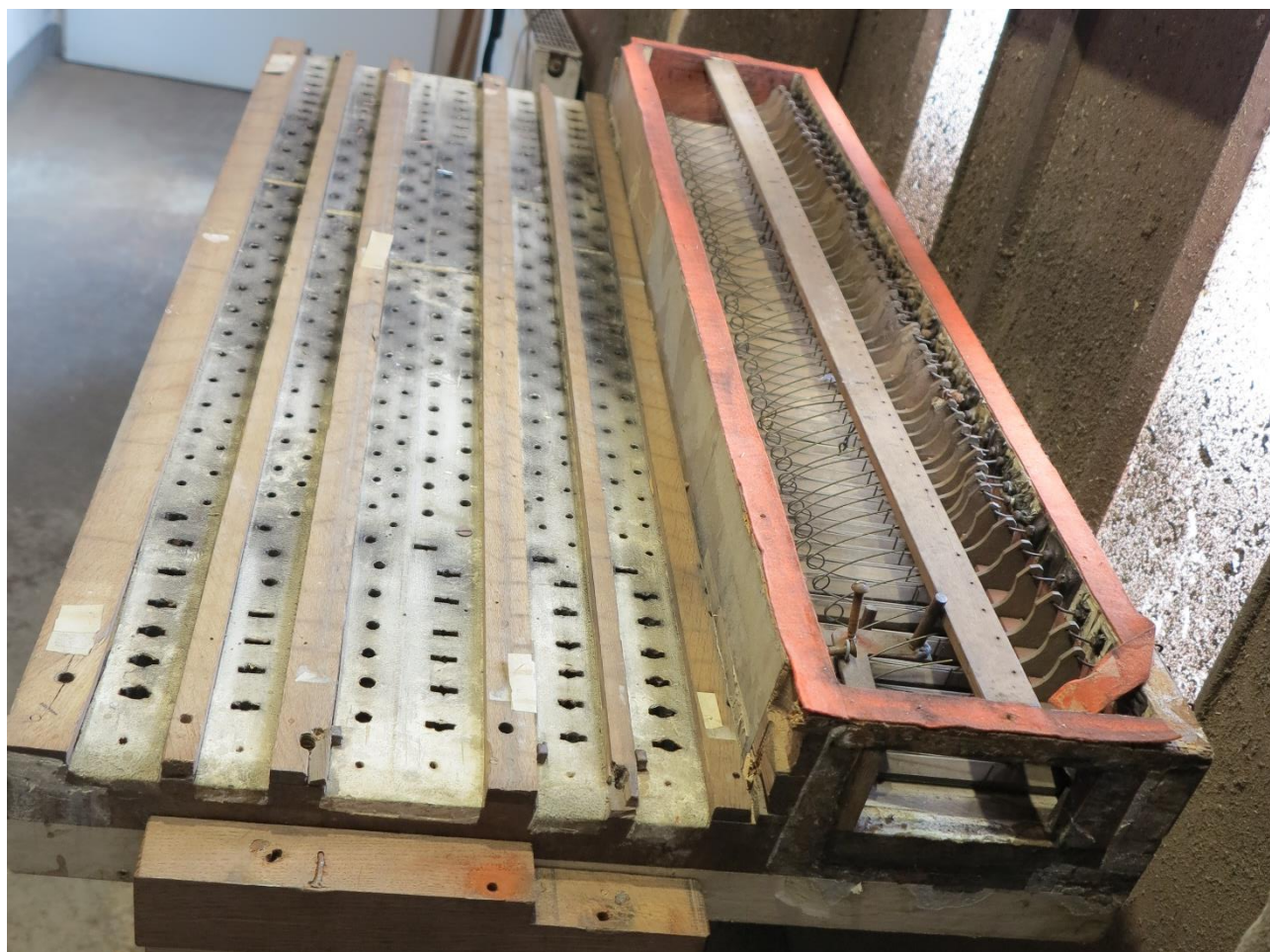
Vzdušnice pozitivu – před demontáží
